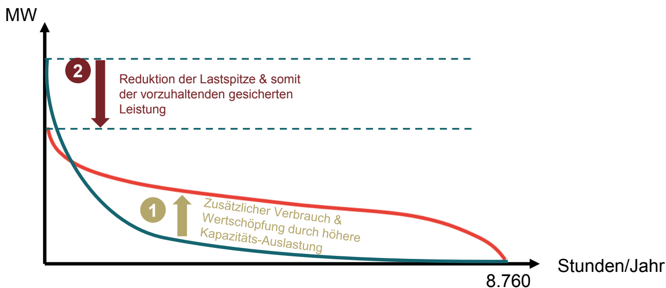
Abbildung 4. Vorteile einer Erschließung der Wertschöpfung- und Flexibilitätpotenziale des Stromverbrauchs am Beispiel einer Lastdauerkurve (schematisch)
